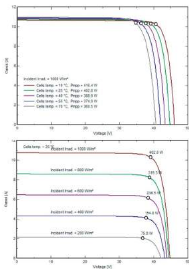
Eigenschaften bei unterschiedlicher Einstrahlung
